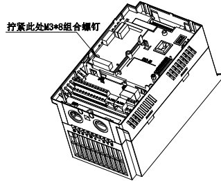
图附 1 I/O 扩展卡安装示意图
